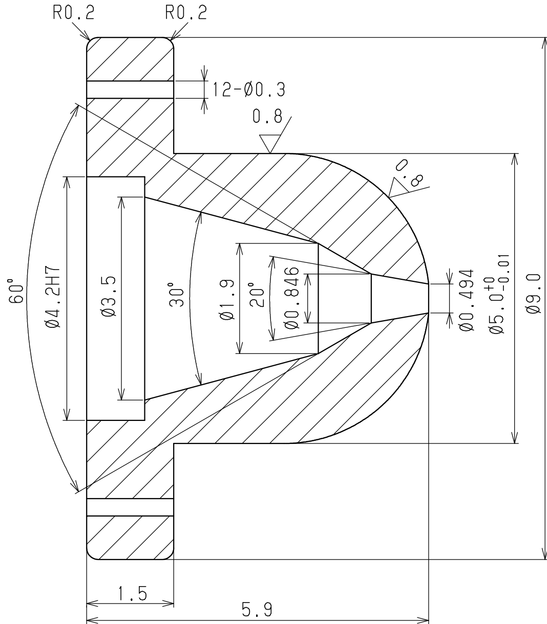
縦断面図
