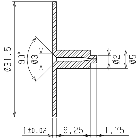
縦断面図
