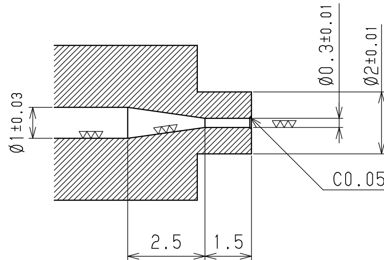
先端拡大図
