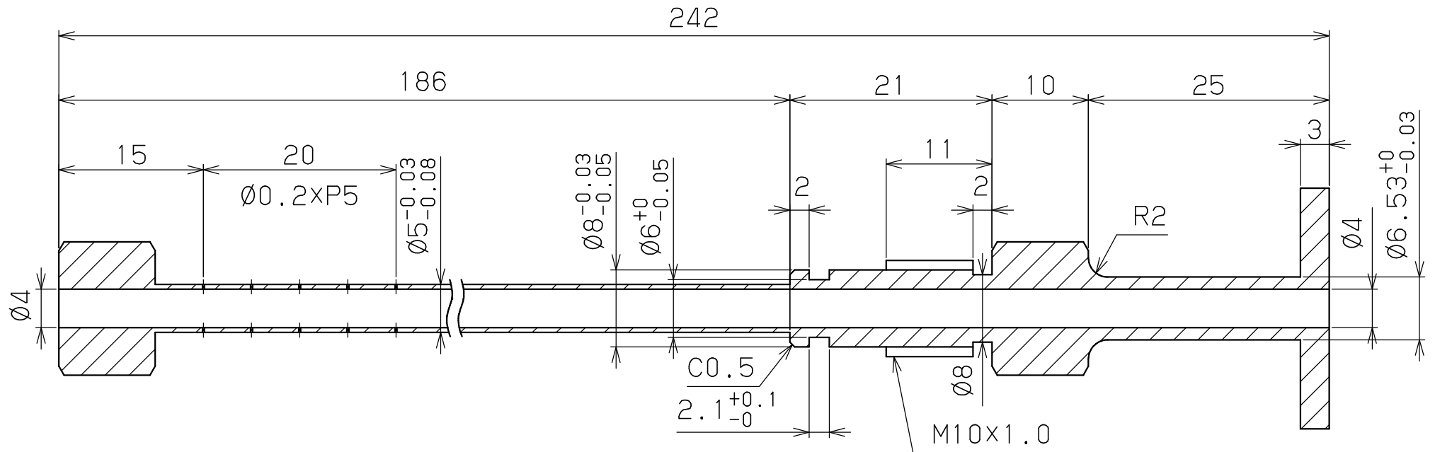
中間省略した縦断面図
