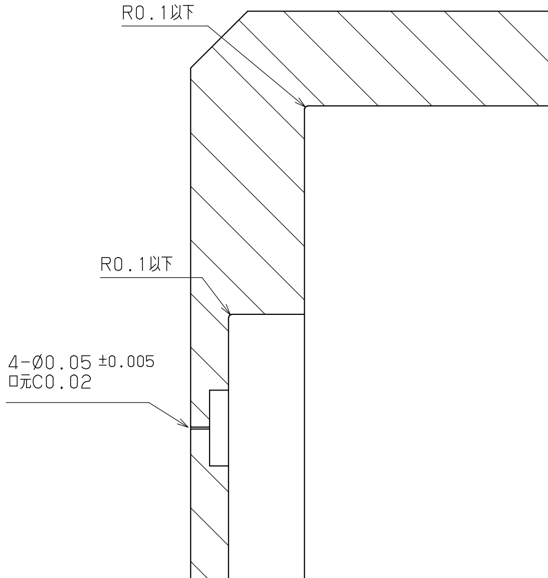
上半分拡大断面図
