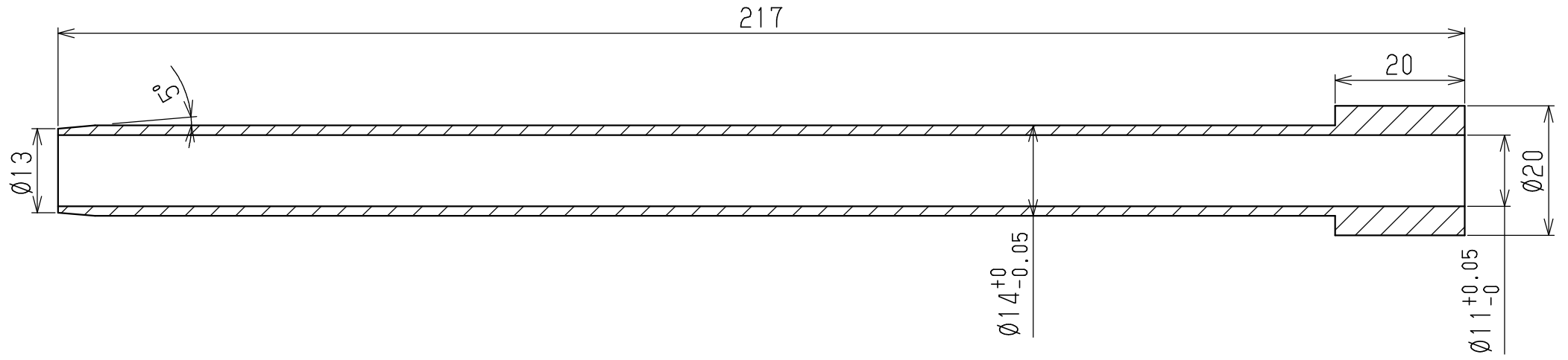
縦断面図
