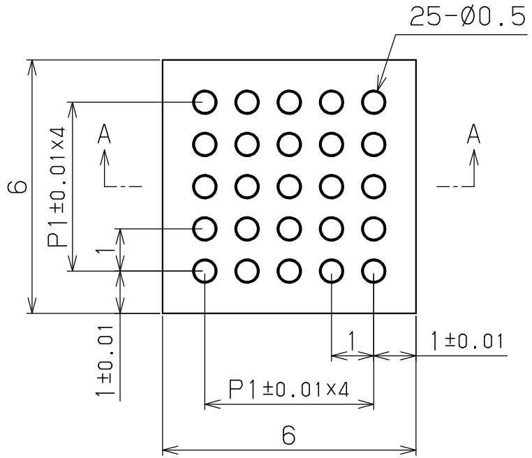
平面図
