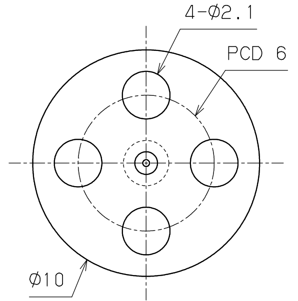
右側面図
