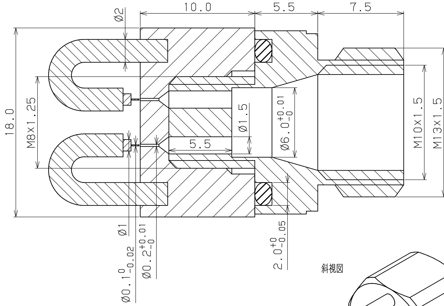
縦断面図
