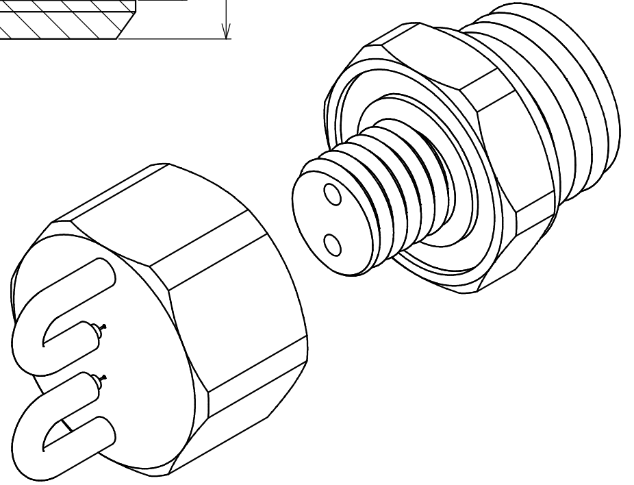
斜視図
