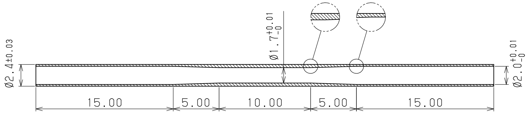
縦断面図
