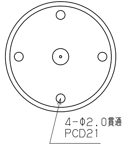
右側面図
