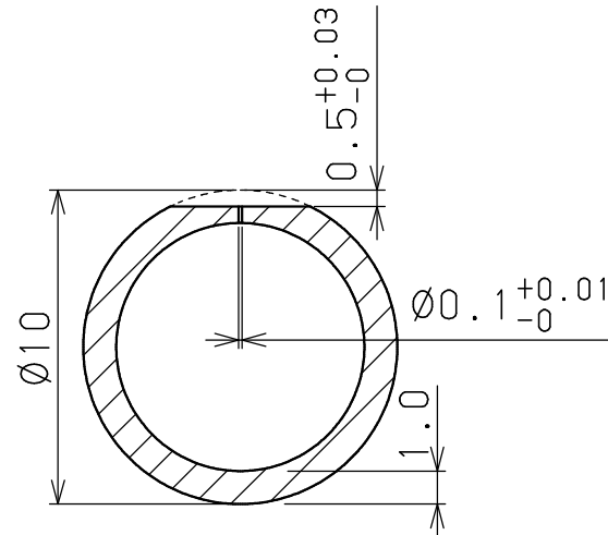
B部拡大断面図
